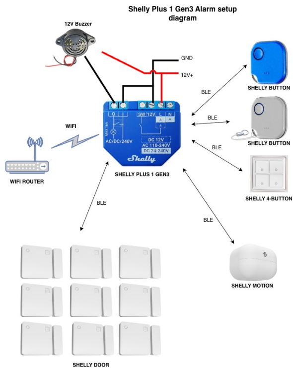
Figure 1 - Sådan ser systemet grundlæggende ud – Der kan tilsluttes urimeligt mange sensorer
